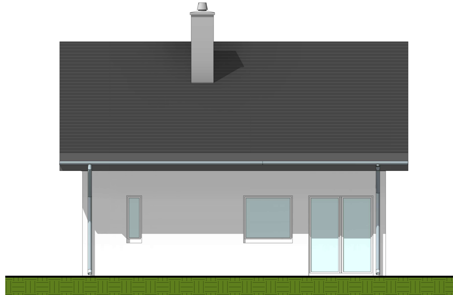
1 Elewacja ogrodowa 1 : 50
